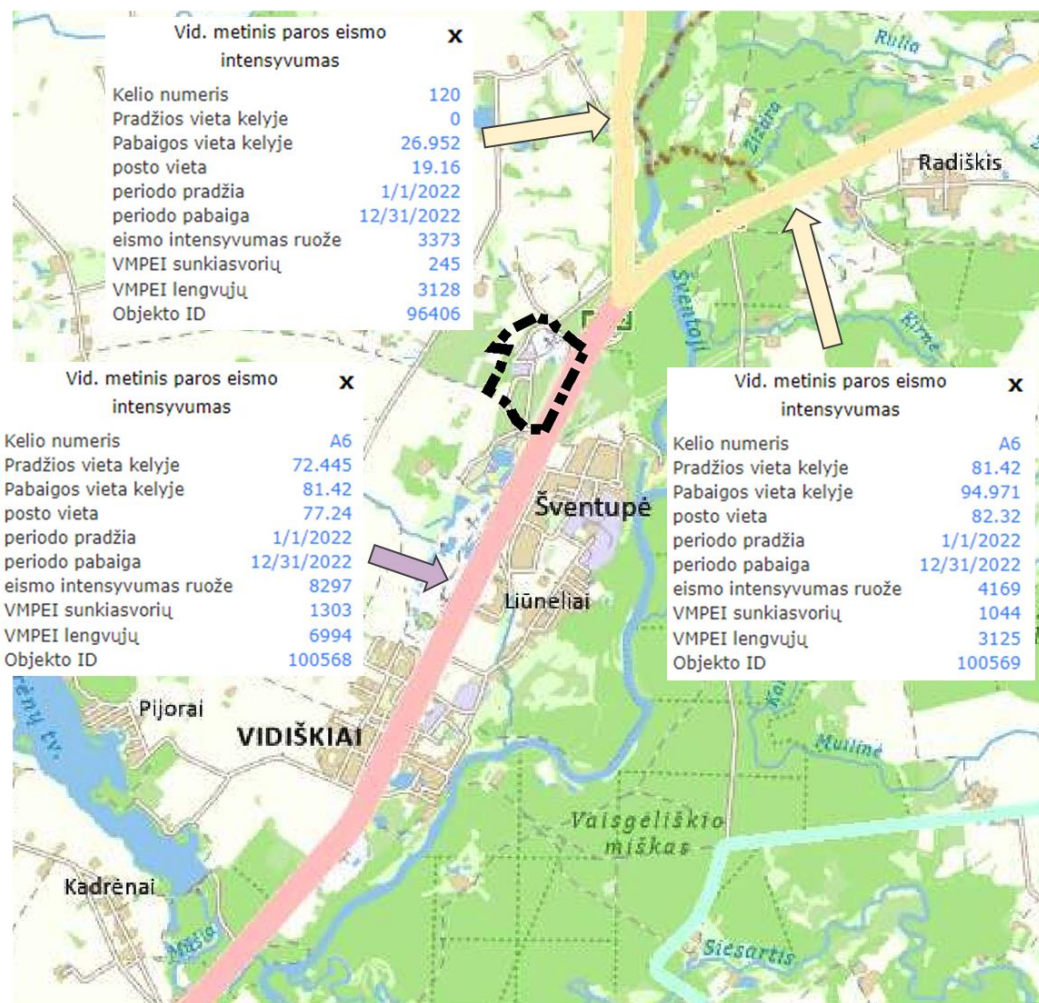
22 pav. Vidutinis metinis paros eismo intensyvumas valstybinės reikšmės keliuose 2022 metais Šaltinis: https://eismoinfo.lt/#/ (schema sudaryta Rengėjo)
